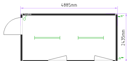
Bürocontainer 16'
