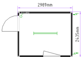
Bürocontainer 10'
